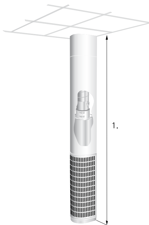
Рис. 5. DHC с декоративным коробом воздуховода и цокольным листом
