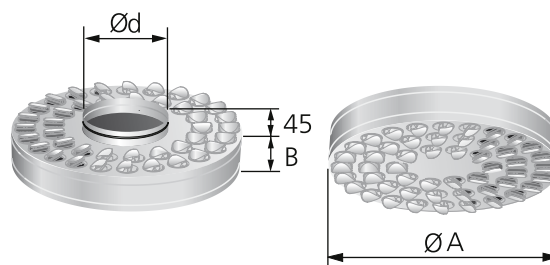
Рис. 2. Диффузор EAGLE Single / Double
