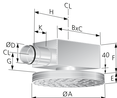
Рис. 3. EAGLE Single / Double с ALS
